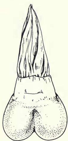
— — — — — Oceanodroma melania
